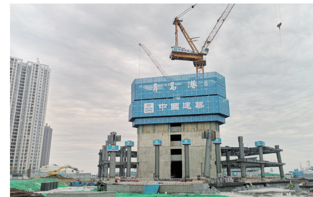
青岛港安置楼项目 Qingdao port resettlement building project
